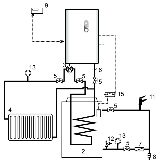
Принципиальная схема подключения бойлера.
